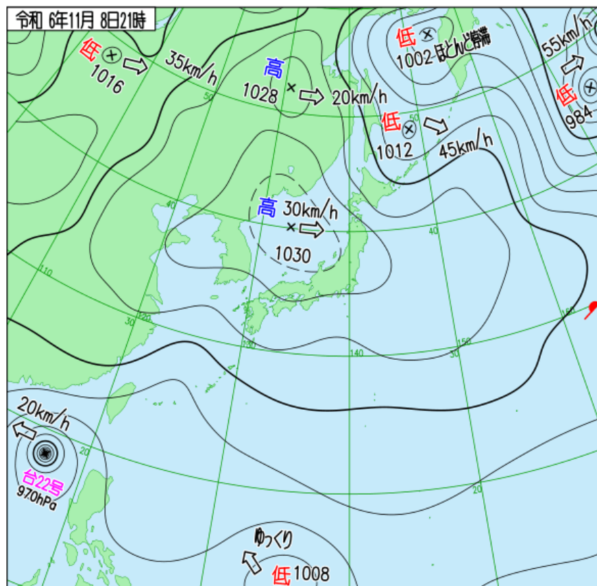
天気図 (11月8日21時)
