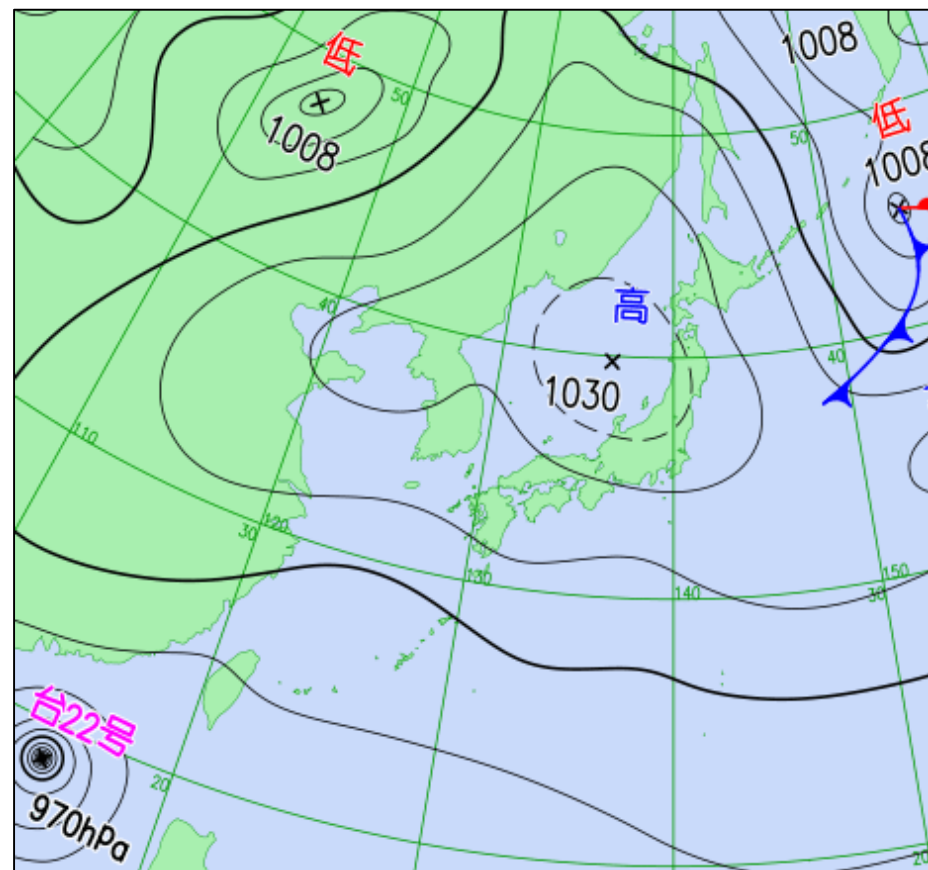
予想天気図 (11月9日09時予想)
