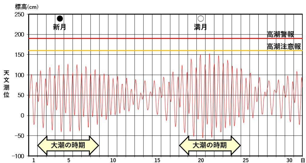
図3 博多における2024年8月（1時間ごとの）の天文潮位
