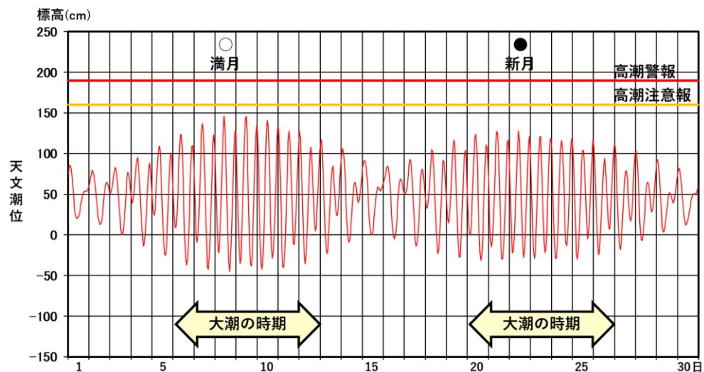
図3 博多における2025年9月（1時間ごとの）の天文潮位
