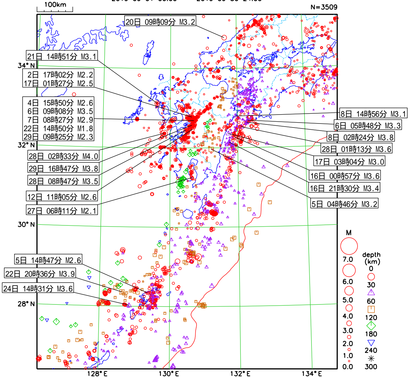
震央分布図（震度1以上を観測した地震に吹き出しを付けた。）
