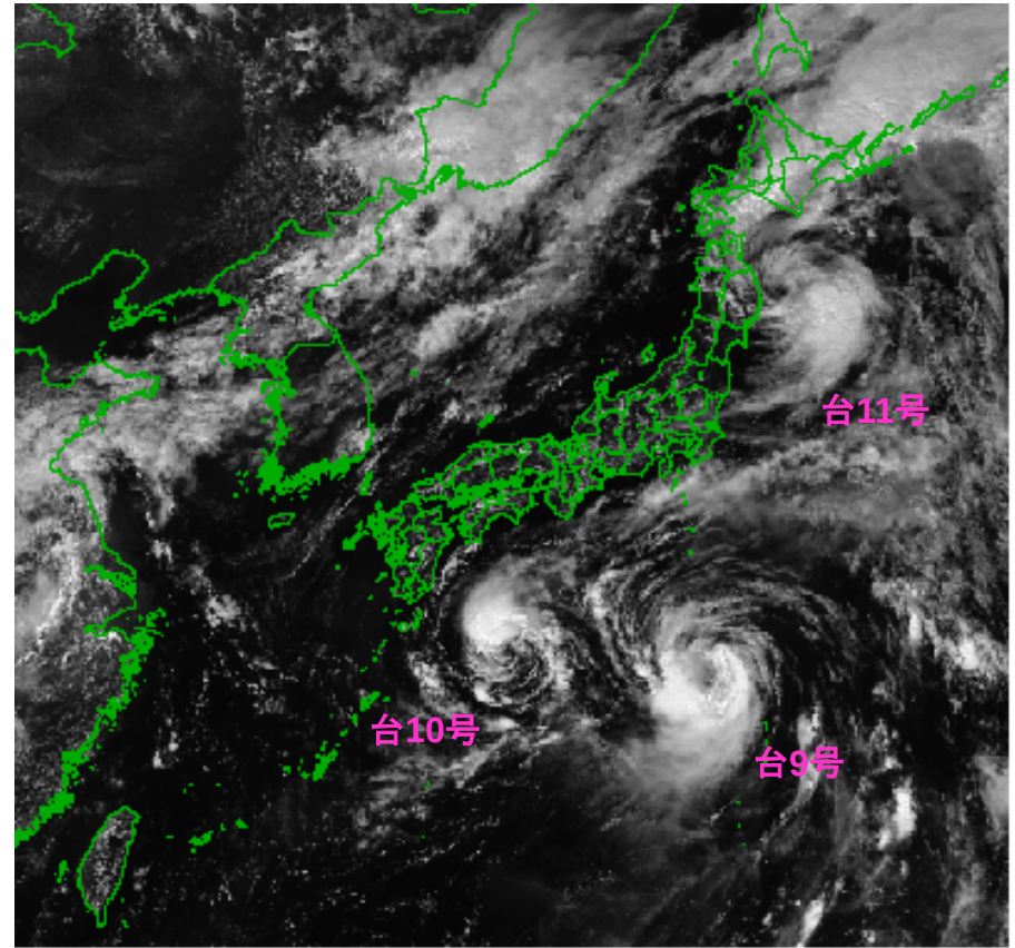
気象衛星画像 (2016年8月21日12時)
