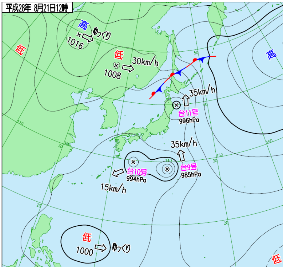
地上天気図 (2016年8月21日12時)
