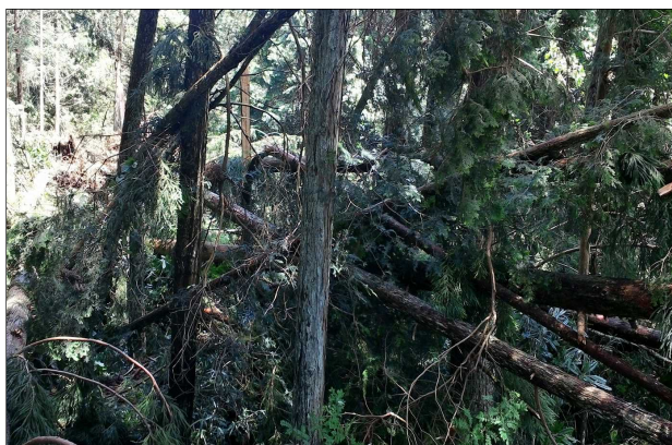
① 幹折れした針葉樹 (南西方向から撮影)
