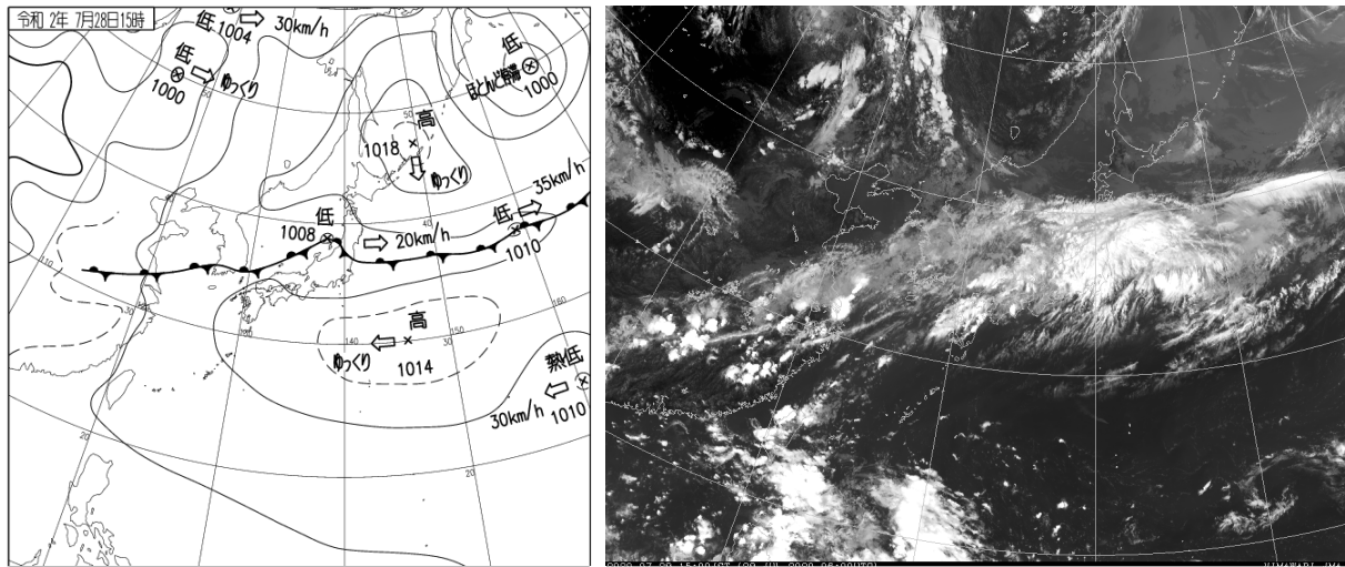
7月28日15時の地上天気図（左）と気象衛星赤外画像（右）
