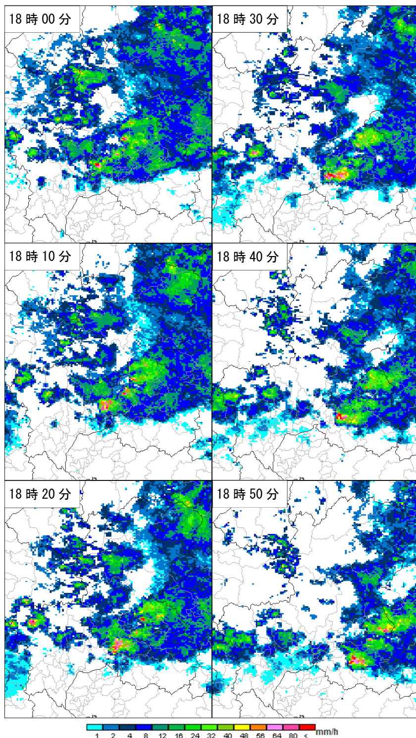
7月28日18時00分から10分毎のレーダー画像
