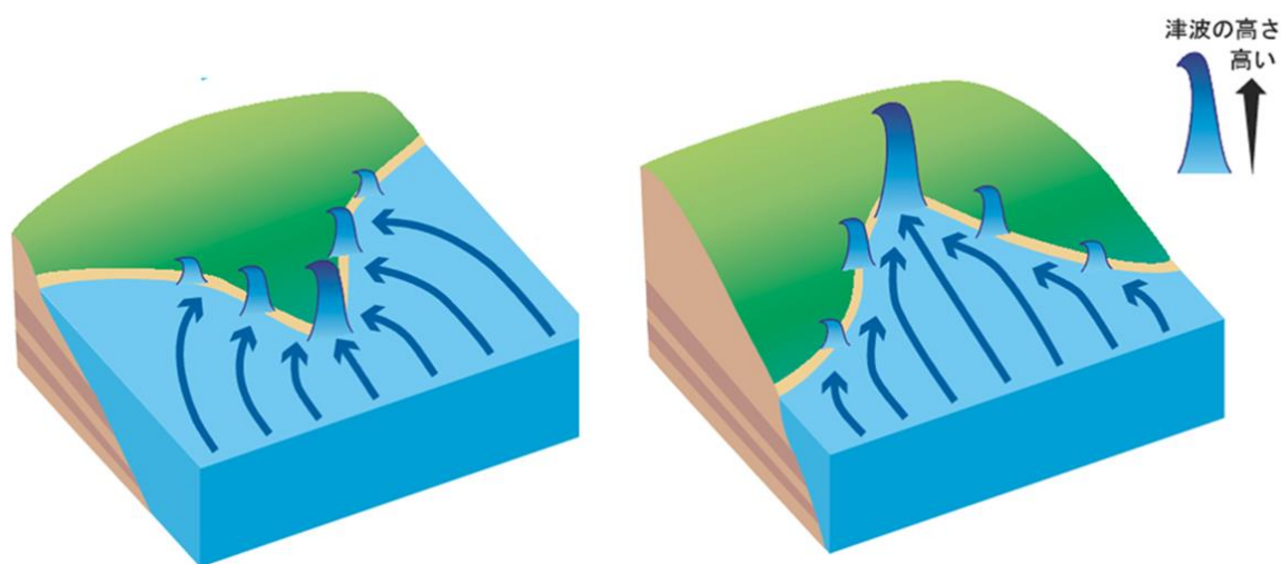
図4 岬の先端やV字型の湾の奥に津波が集まる様子
