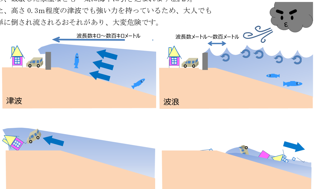
図2 津波と波浪の違い
