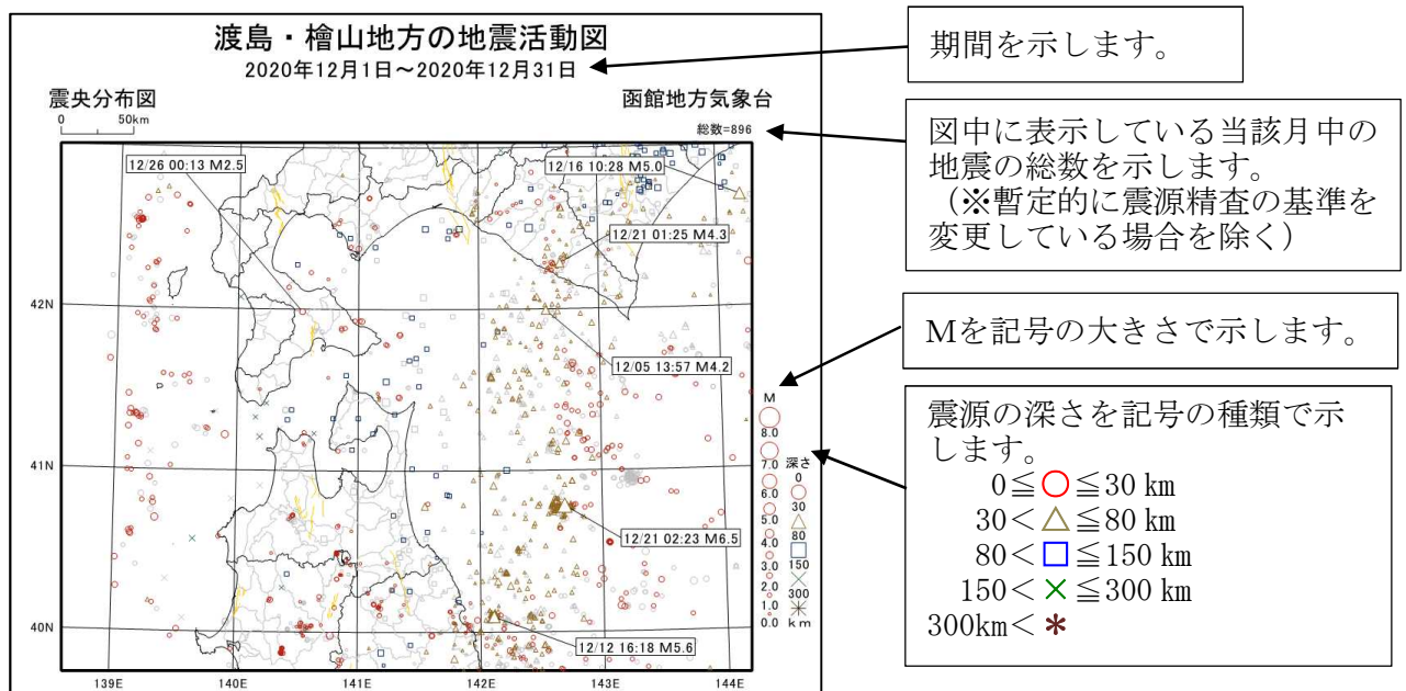
図1 震央分布図
