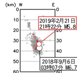
図6 断面図の例
