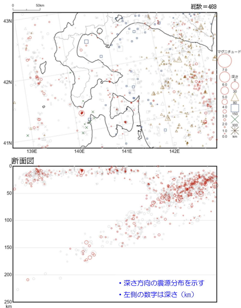
図２ 断面図の例
