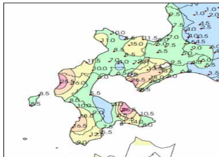
1時間雨量の最大値
