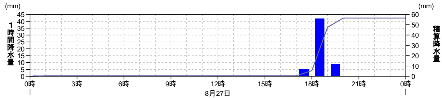
■ 8月27日の1時間降水量と積算降水量(1時間ごと)
