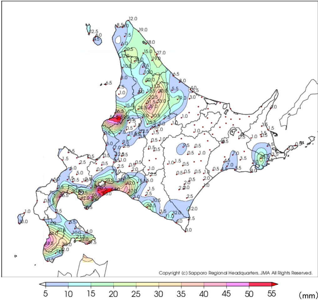
8月27日の日降水量の分布図と一覧表(上位20地点)
