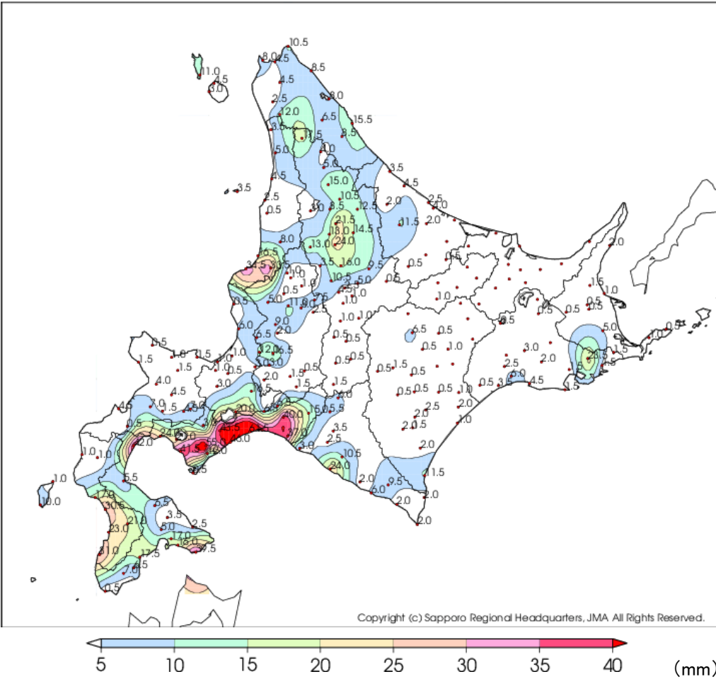
8月27日の最大1時間降水量の分布図と一覧表(上位20地点)
