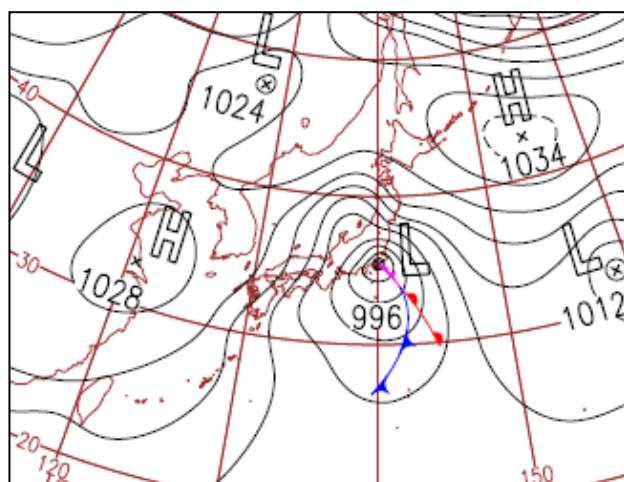
第1図 2014年2月15日09時 地上天気図 ※羽田で13cmの降雪を記録した日
