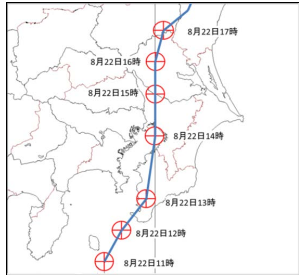
第 7 図 台風第 9 号経路図
