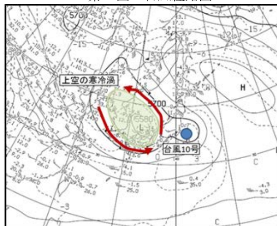
第4図 500h pa 面天気図 (8月30日9時JST)
