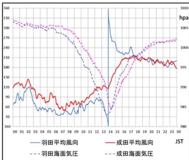
第9図 8月22日羽田空港・成田空港 風向と海面気圧
