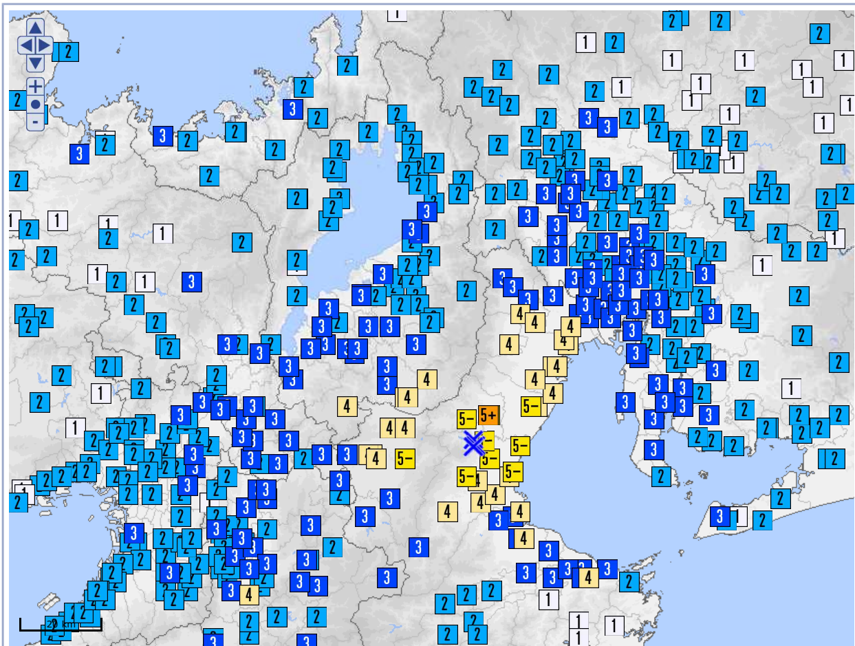
震度分布図
