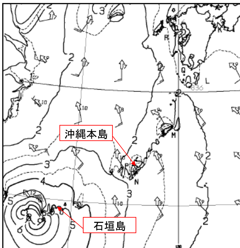
沿岸波浪実況図 2016年9月17日09時 (単位：メートル)
