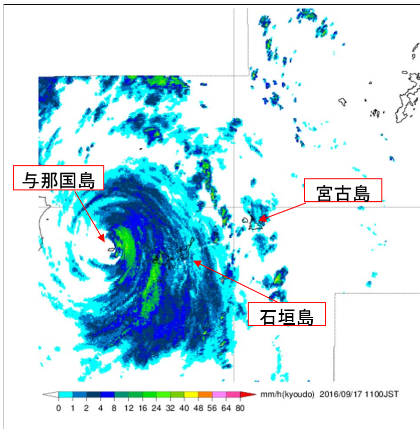
気象レーダー（降水強度）2016年9月17日11時
