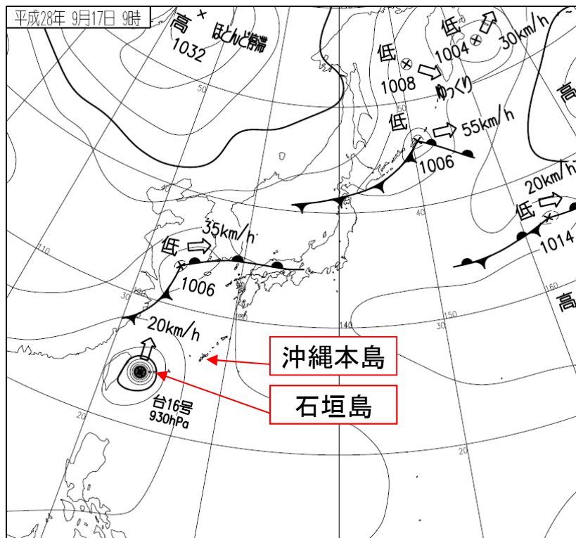
地上天気図 2016年9月17日09時
