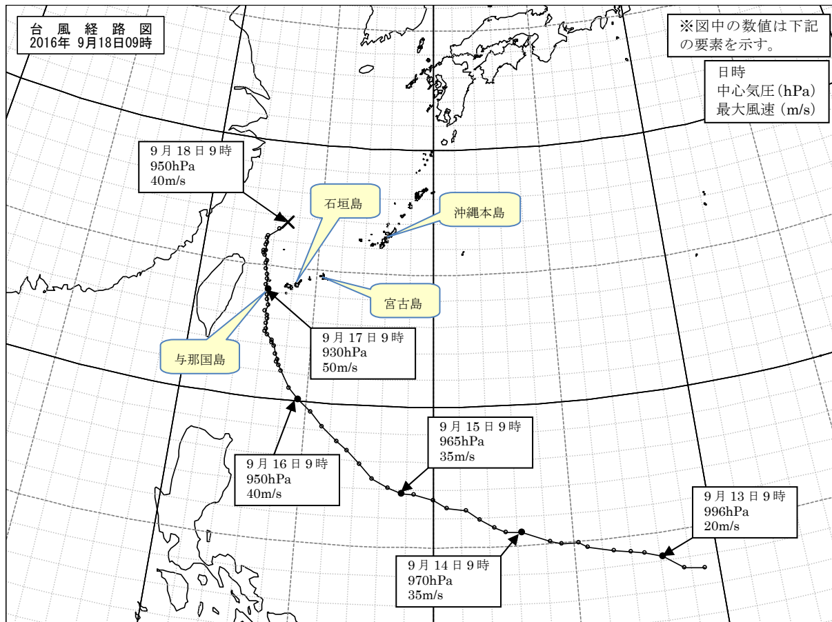
台風第16号経路図 (2016年9月18日09時現在 速報値)
