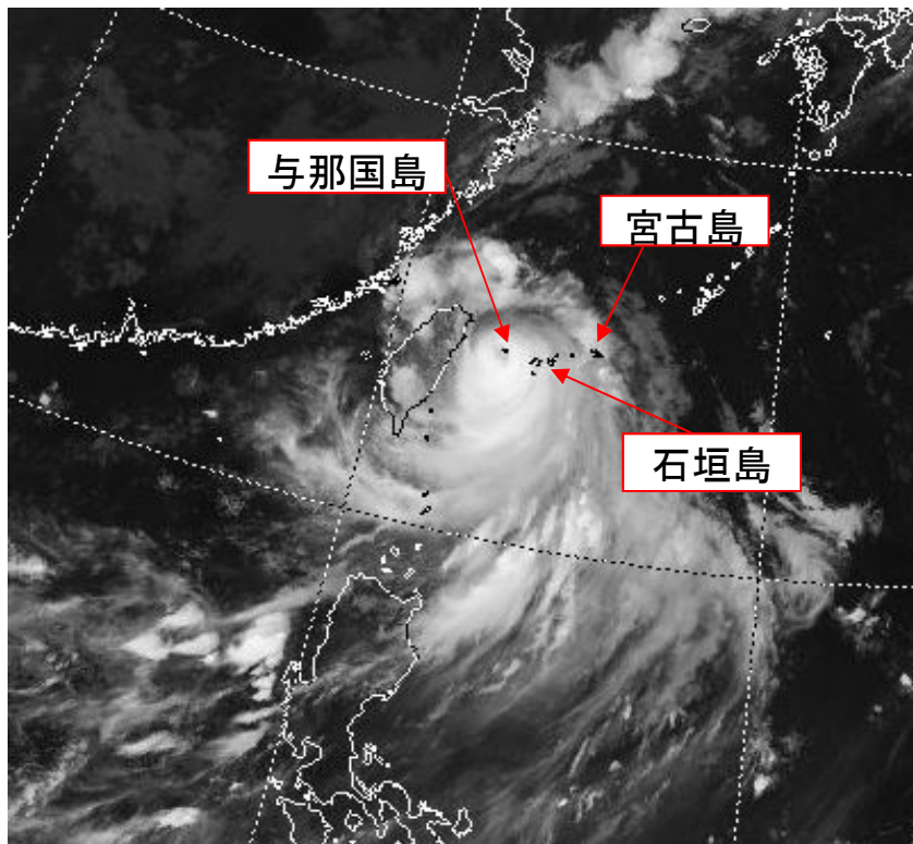
気象衛星画像（赤外）2016年9月17日11時
