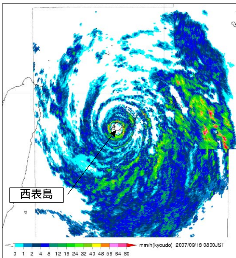
レーダーエコー図 平成19年9月18日08時00分
