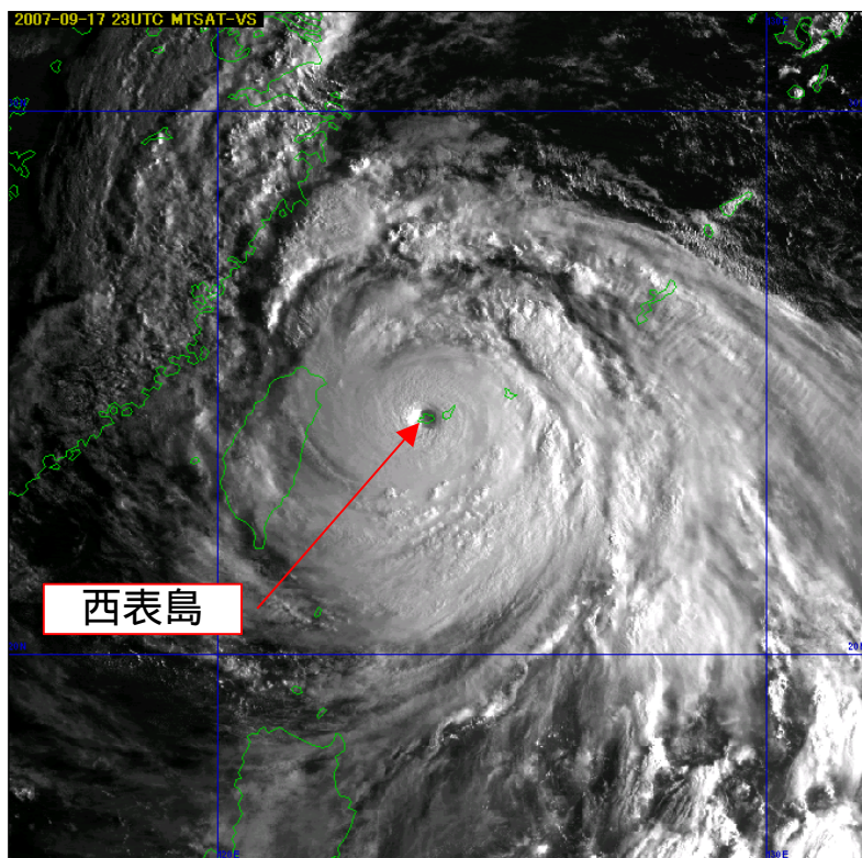
気象衛星画像（可視）平成19年9月18日08時
