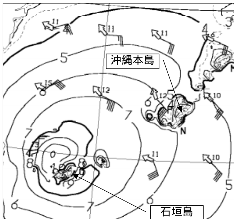
沿岸波浪実況図 平成19年9月18日09時
