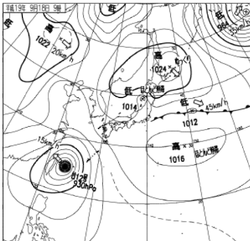
地上天気図 平成19年9月18日09時
