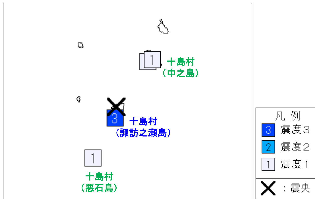
震度分布図(観測点別) 9月21日05時34分 M3.8
