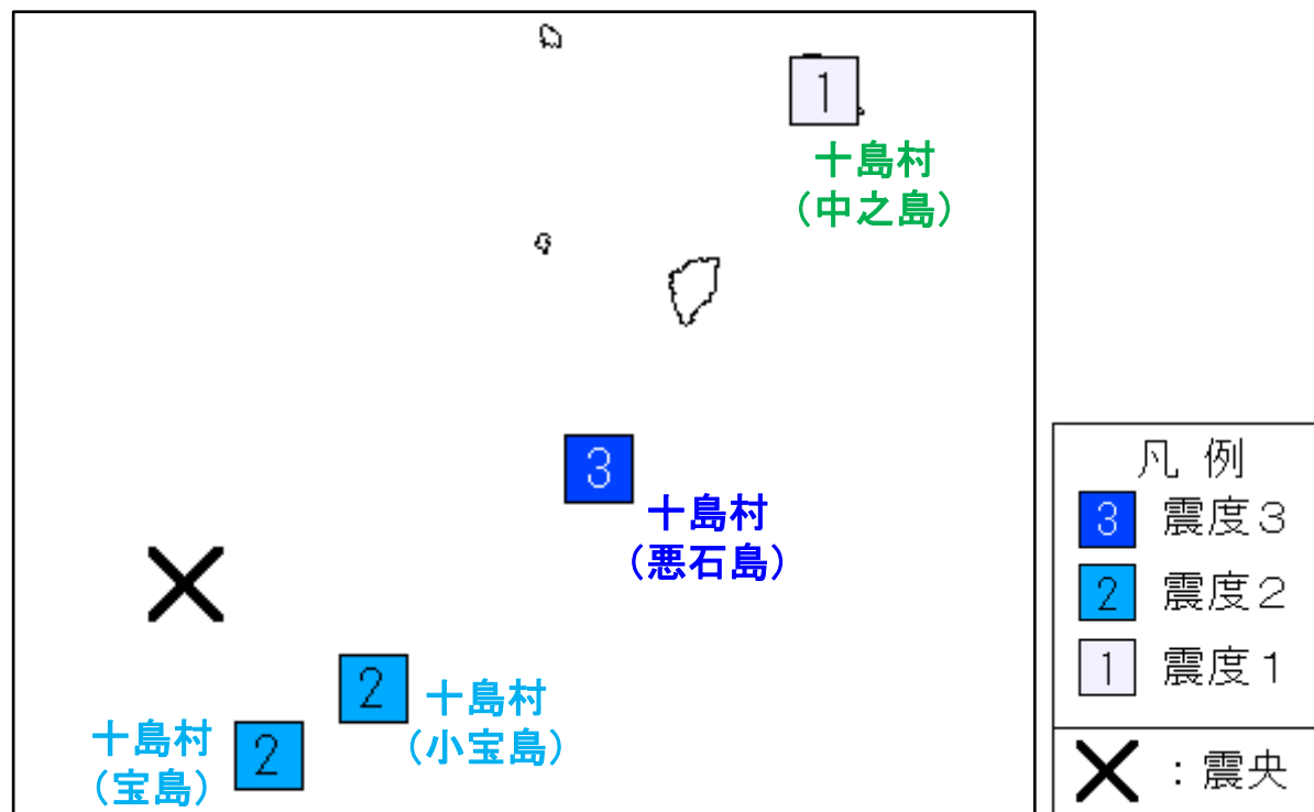
震度分布図(観測点別) 10月8日06時38分 M5.3
