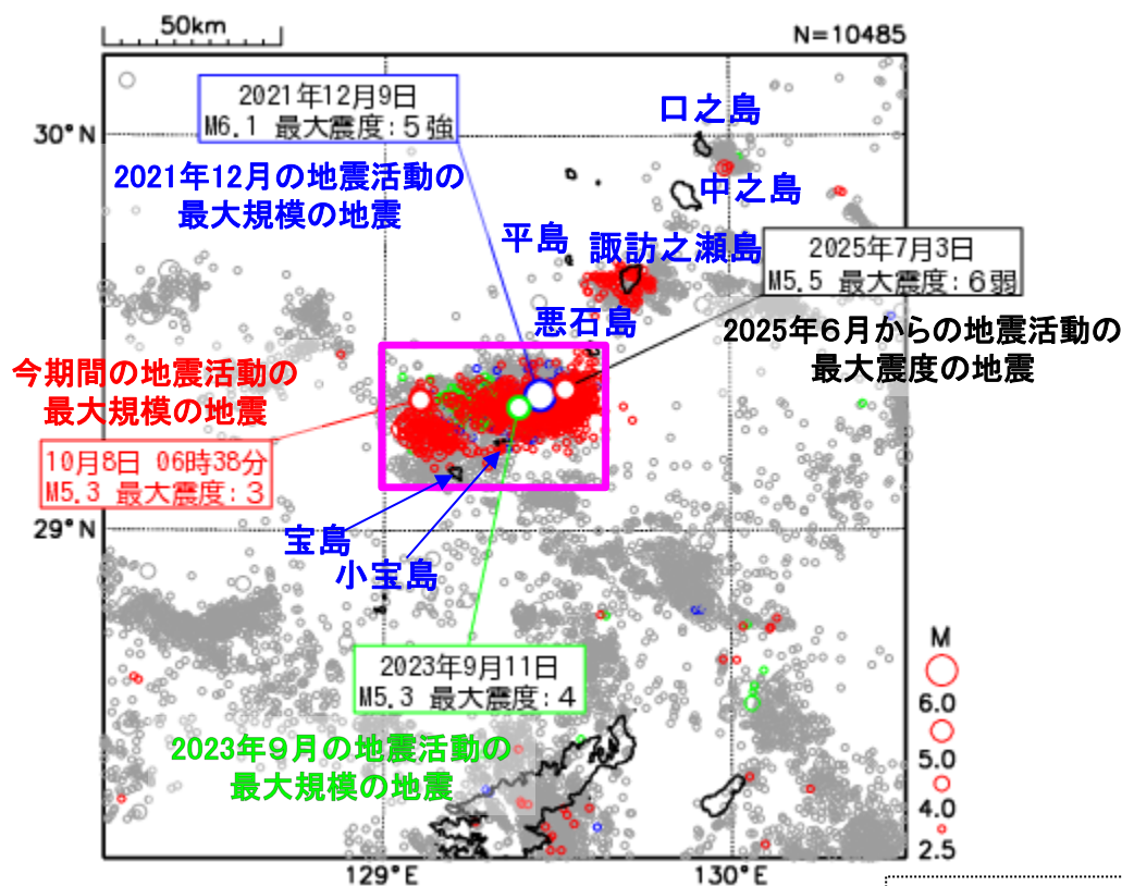
震央分布図 (1994年10月1日～2025年10月19日、 M \geq 2.5 、深さ0～40km)
