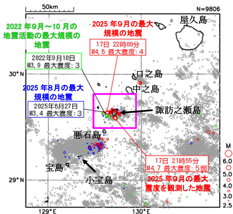
震央分布図
