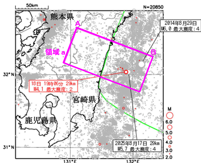
震央分布図
