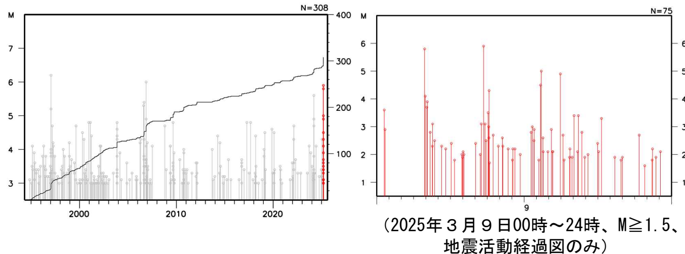
領域a内の地震活動経過図及び回数積算図
