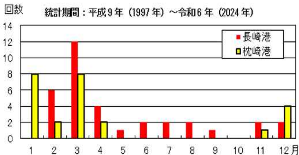
図2 「あびき」の月別発生回数 （長崎港（長崎県）と枕崎港（鹿児島県）における100センチ以上の回数）
