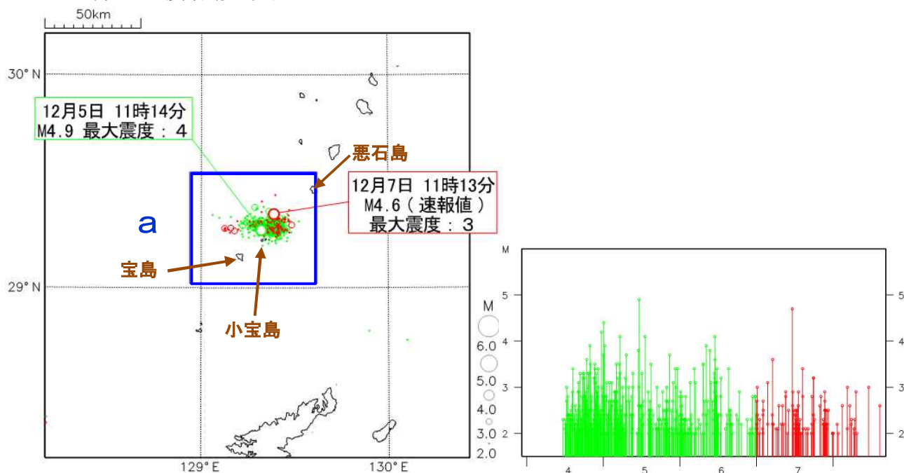
震央分布図
