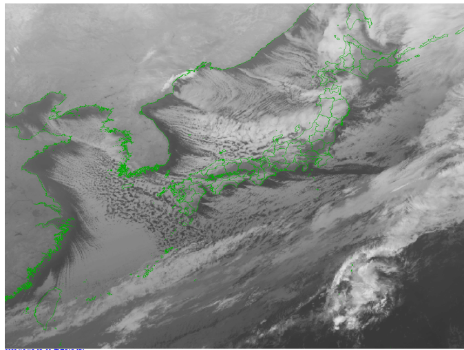
12月18日09時の地上天気図（左）と気象衛星赤外画像（右）
