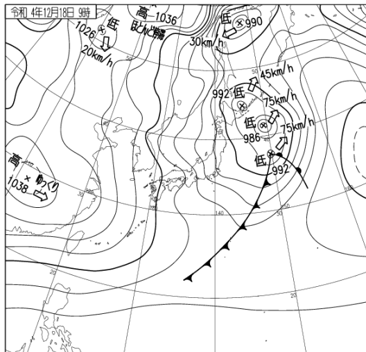
12月18日09時の地上天気図（左）と気象衛星赤外画像（右）
