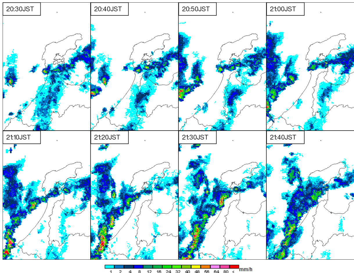
10月19日20時30分から10分毎のレーダー画像
