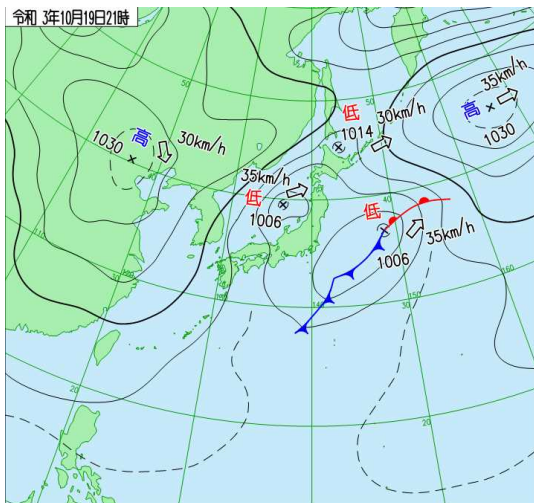
10月19日21時の天気図
