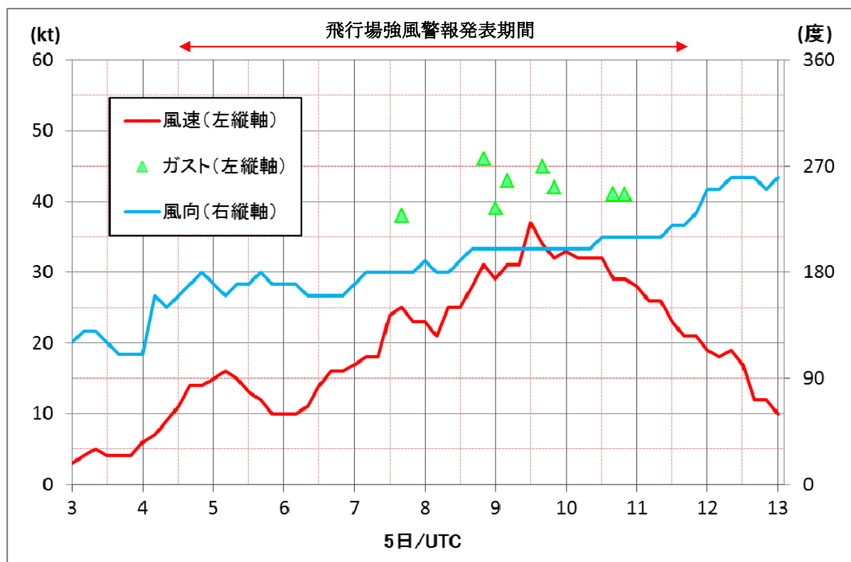
第 3 図 関西国際空港代表風 (06R) の風向と風速 (5 日 03UTC~13UTC)
