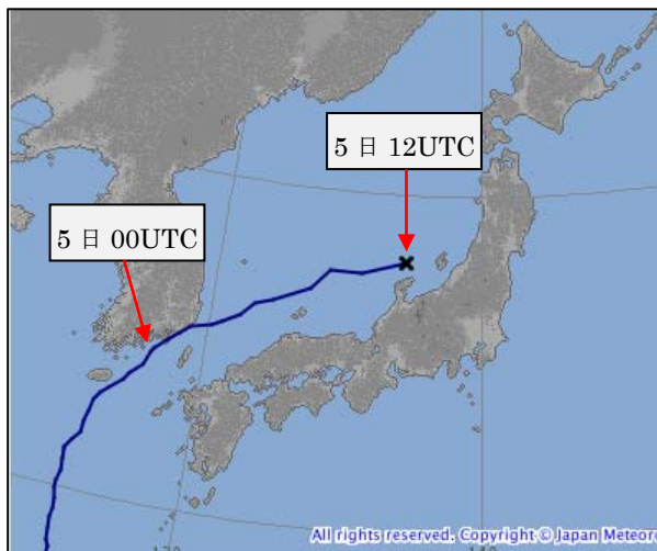
第 2 図 台風経路図
