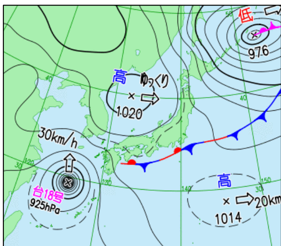
第 1 図 速報天気図（10 月 4 日 06UTC）
