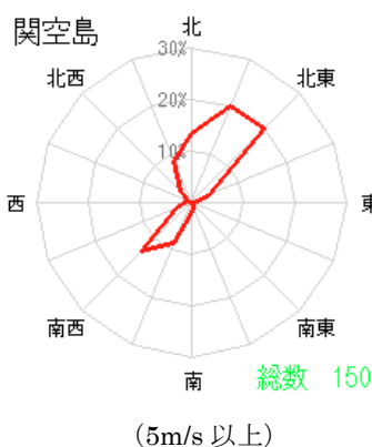
第4図 2024年4月の風速階級別風配図
