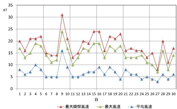
第2図 2024年4月の日別風速
