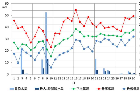
第1図 2024年4月の日別気温・降水量
