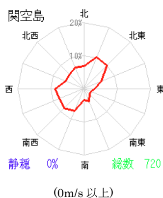
第3図 2024年4月の風配図
