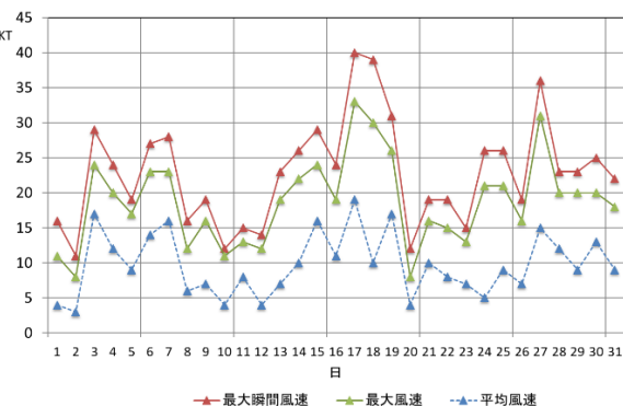
第2図 2025年3月の日別風速
