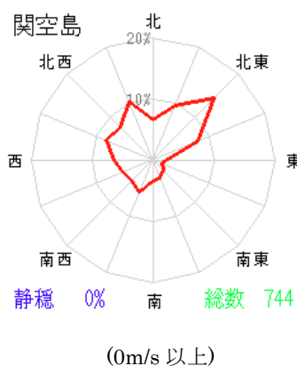
第3図 2025年3月の風配図
