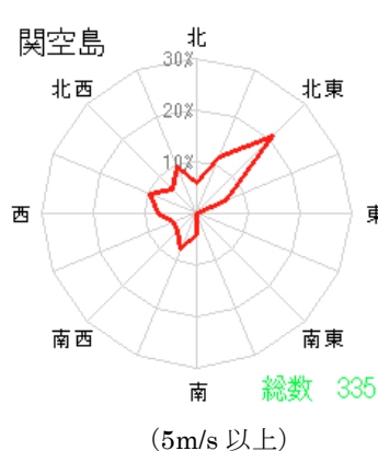
第4図 2025年3月の風速階級別風配図
