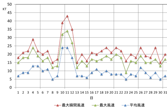
第2図 2025年8月の日別風速
