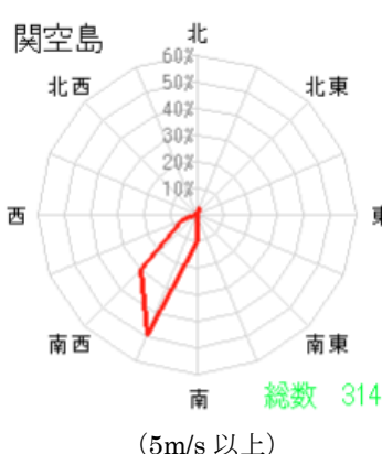
第4図 2025年8月の風速階級別風配図
