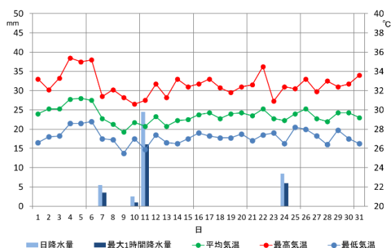
第1図 2025年8月の日別気温・降水量
