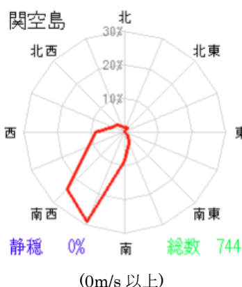
第3図 2025年8月の風配図
