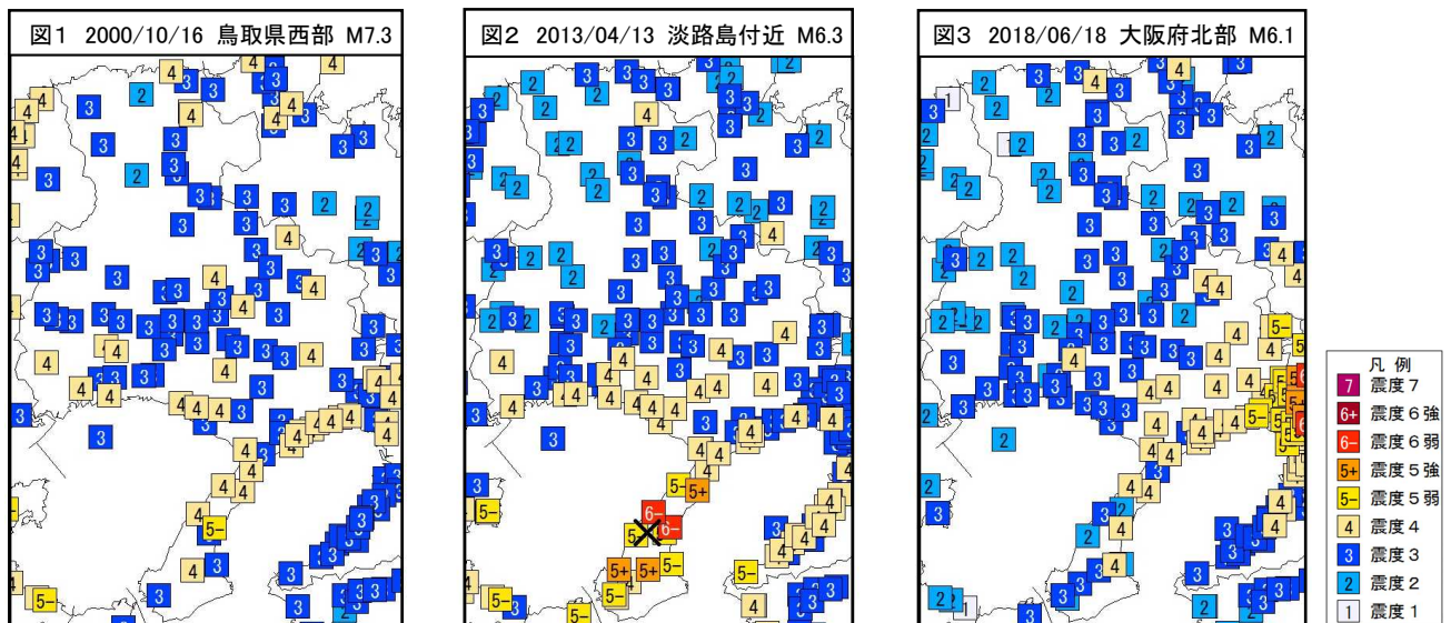
図1～3 兵庫県内で震度5弱以上を観測した地震の県内震度分布図
