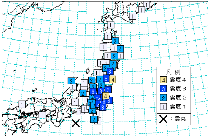
図1 地域震度分布図
