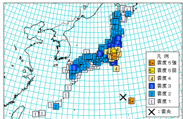
図3 地域震度分布図 2015年5月30日の小笠原諸島西方沖の地震
