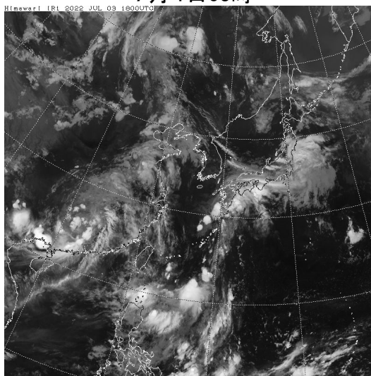
気象衛星赤外画像 7月4日03時
