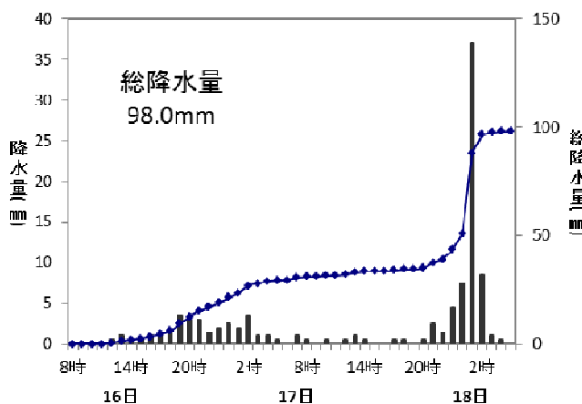
古関（山梨県甲府市）
