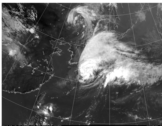
気象衛星赤外面像 (9月17日15時)
