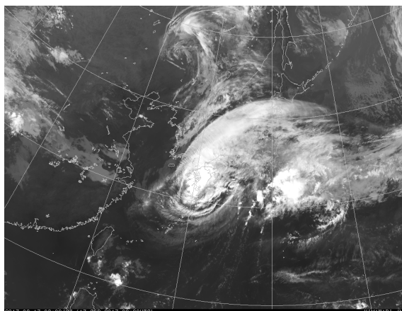
気象衛星赤外面像 (9月17日09時)
