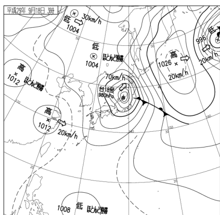
地上天気図 (9月18日03時)
