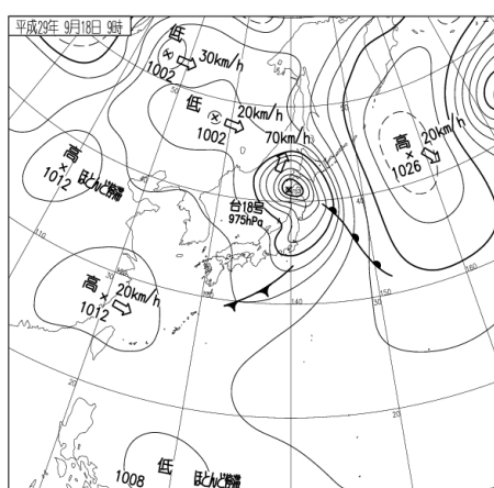
地上天気図 (9月18日09時)
