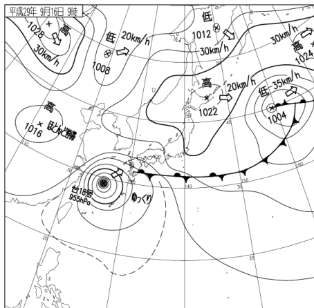
地上天気図 (9月16日09時)
