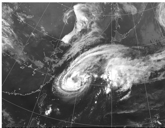
気象衛星赤外面像 (9月17日03時)
