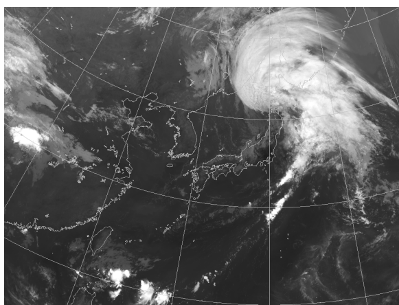
気象衛星赤外面像 (9月18日09時)
