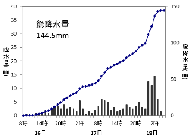
古関（山梨県甲府市）
