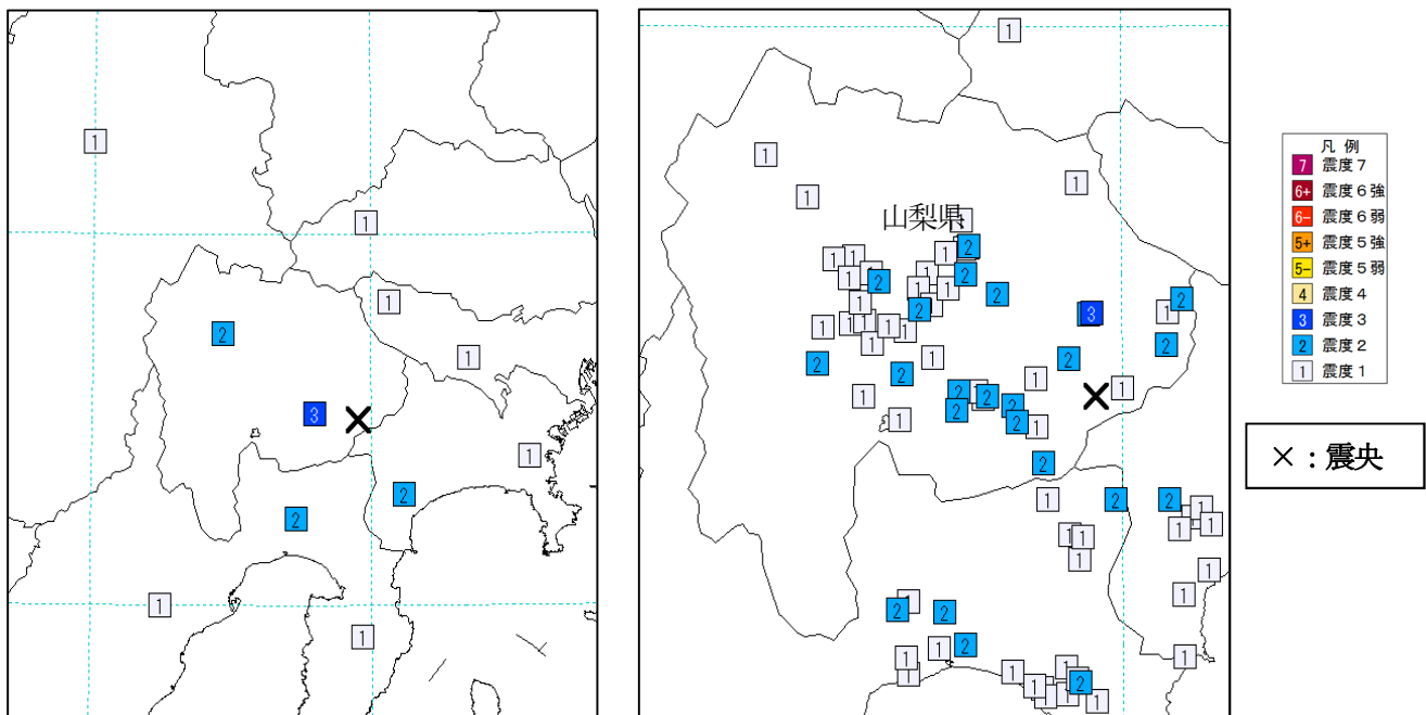
図 1 震度分布図（5 日 08 時 51 分 左図：地域別震度 右図：観測点別震度）
