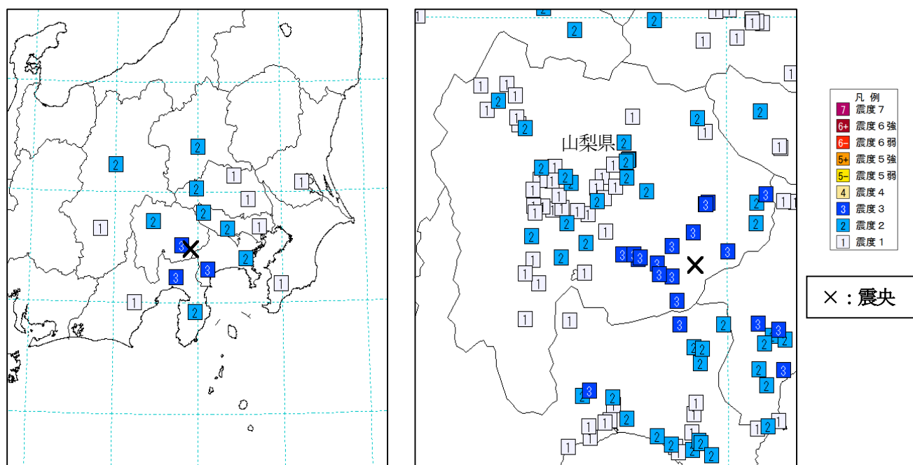
図 1 震度分布図（20 日 22 時 13 分 左図：地域別震度 右図：観測点別震度）
