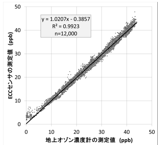
図13 ECCセンサと地上オゾン濃度計の比較図
