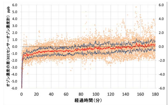
図12 オゾン濃度の差の時間変化
