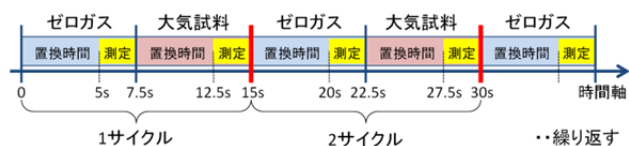
図3 地上オゾン測定シーケンス
