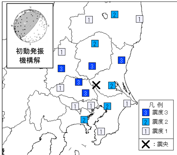
震度分布図
