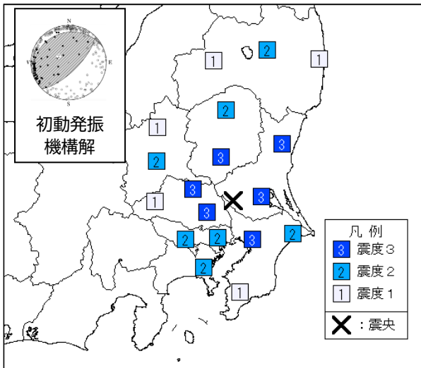
震度分布図
