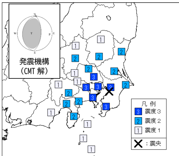
震度分布図
