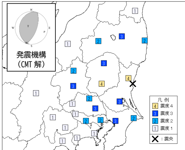
震度分布図
