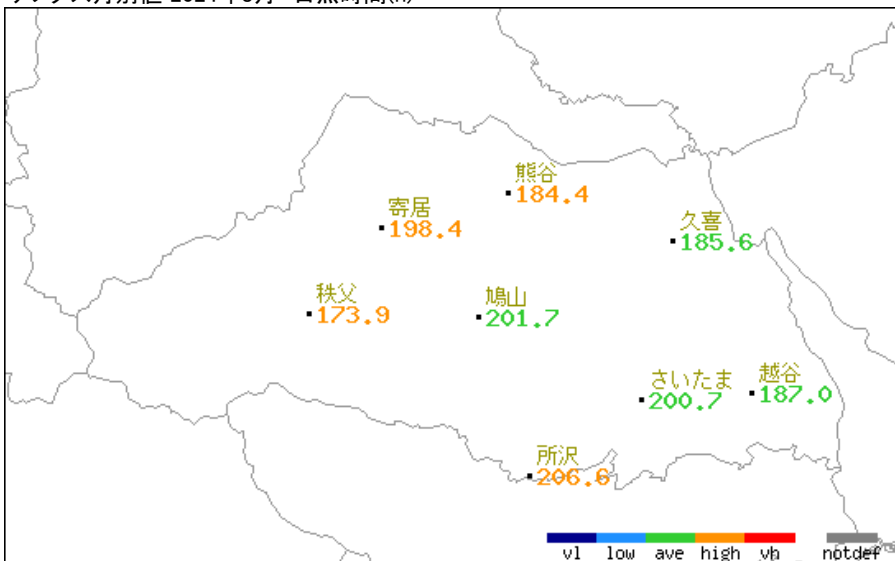
アメダス月別値 2024年8月 日照時間(h)
