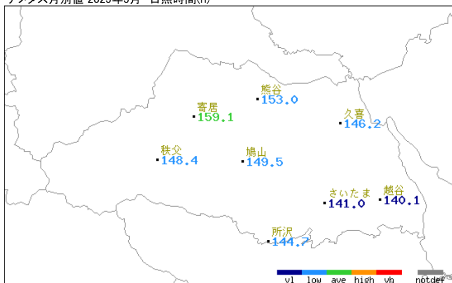
アメダス月別値 2025年5月 日照時間(h)
