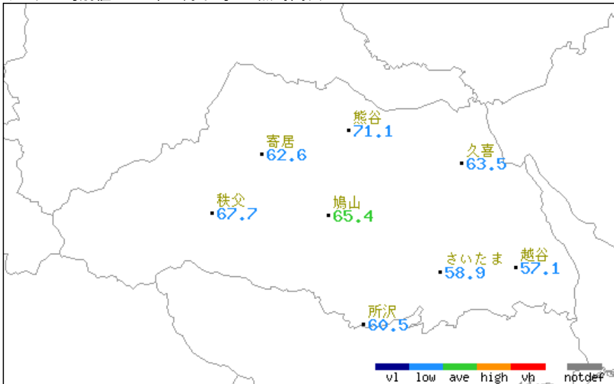
アメダス旬別値 2025年12月下旬 日照時間(h)
