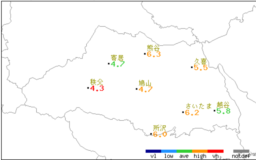
アメダス旬別値 2025年12月下旬 降水量(mm)
