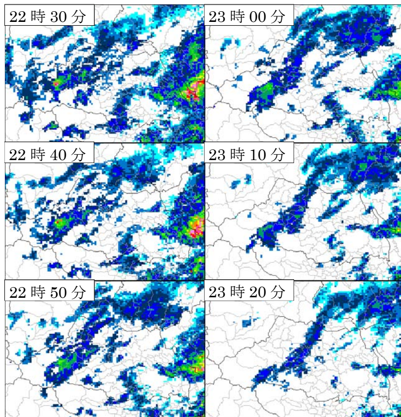
7月4日22時30分から10分毎のレーダー画像
