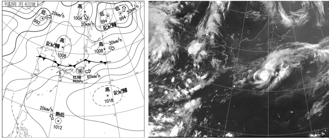
7月4日21時の地上天気図（左）と気象衛星赤外画像（右）
