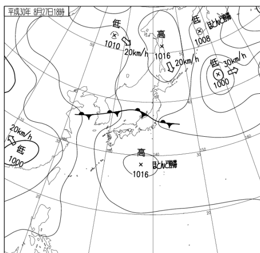
8月27日18時の地上天気図（左）と気象衛星赤外面像（右）
