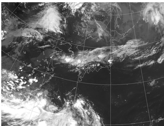
8月27日18時の地上天気図（左）と気象衛星赤外面像（右）
