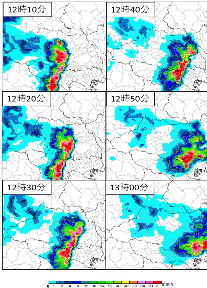
7月24日12時10分から10分毎のレーダー画像
