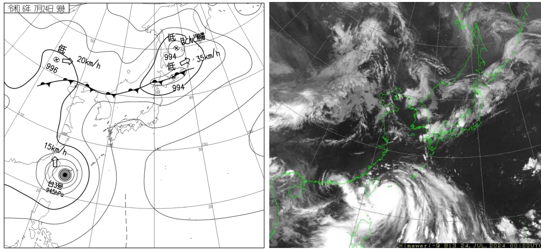
7月24日09時の地上天気図（左）と気象衛星赤外画像（右）
