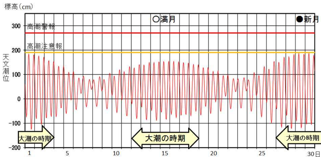
図3 荅北における2019年9月の天文潮位
