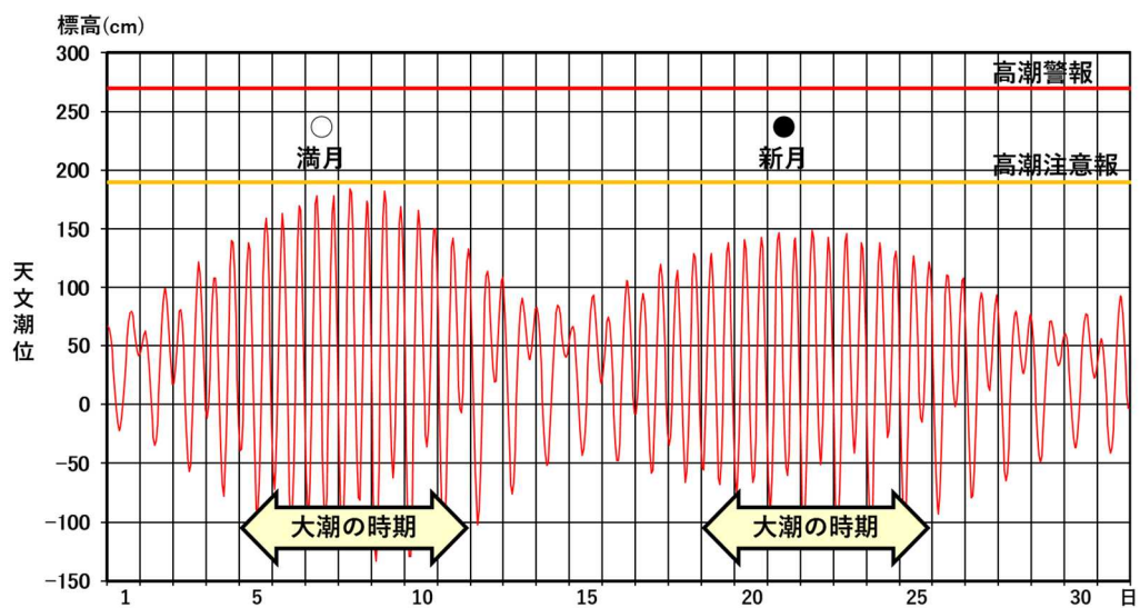
図3 苓北における2025年10月（1時間ごとの）の天文潮位
