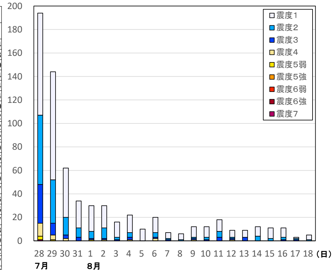
【日別地震回数グラフ】
