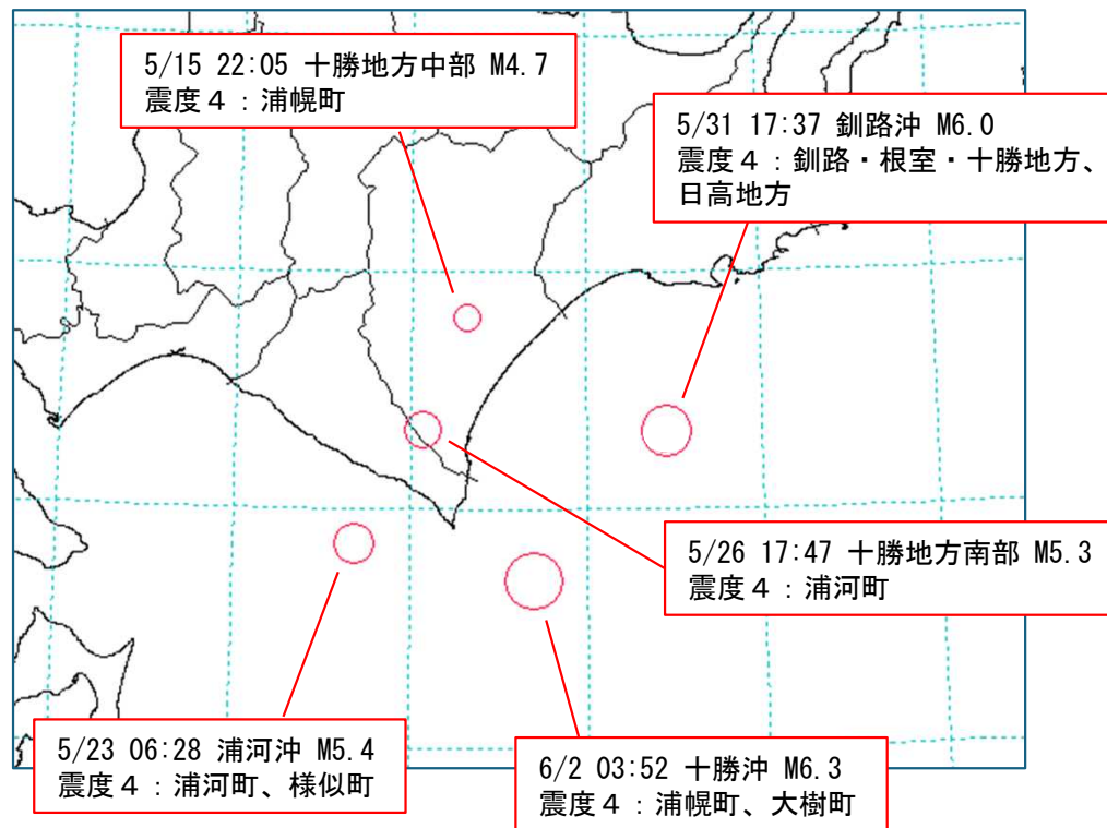
震央分布図（2025年5月以降、最大震度4）
