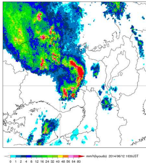
気象レーダー画像（6 月 12 日 16 時 30 分）
