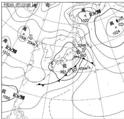
6 月 12 日 15 時（日本時間）の地上天気図
