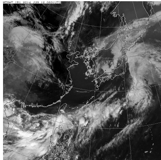
6 月 12 日 16 時（日本時間）の気象衛星赤外画像
