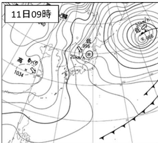
地上天気図(左)と気象衛星赤外画像(右)(2月10日及び11日09時)
