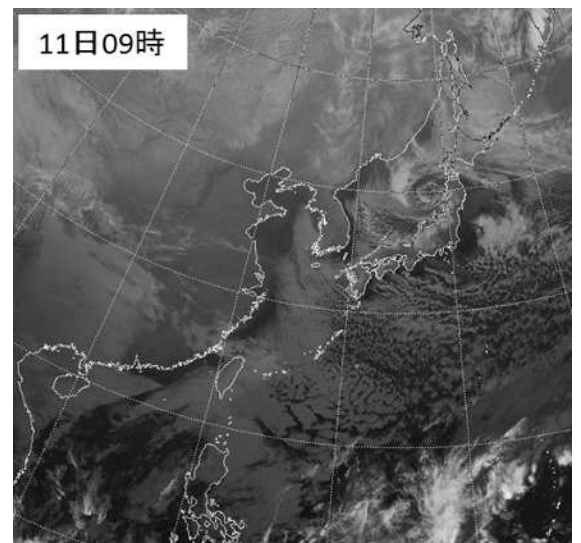
地上天気図(左)と気象衛星赤外画像(右)(2月10日及び11日09時)
