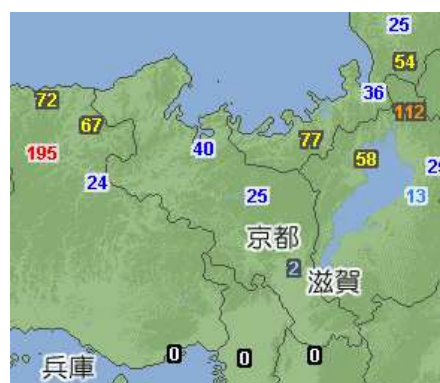
2月11日09時 積雪深 (cm)
