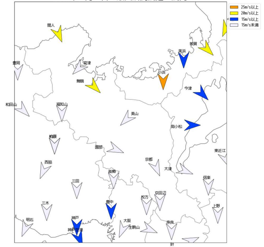
2019年10月13日の最大瞬間風速・風向
